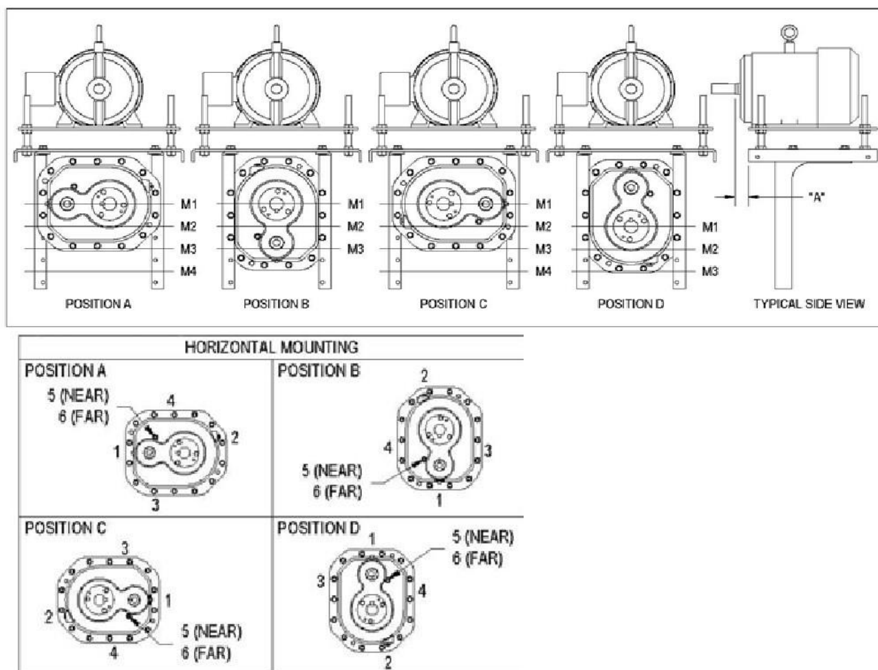
Рис. 6. Рабочие позиции редуктора
